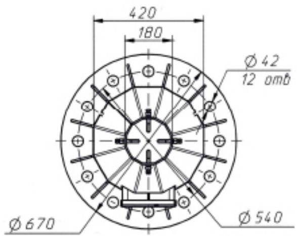
Вид Сверху (1:10)
